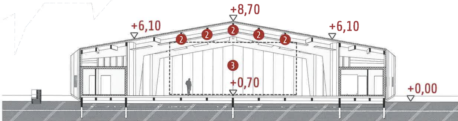
Längsschnitt aa
